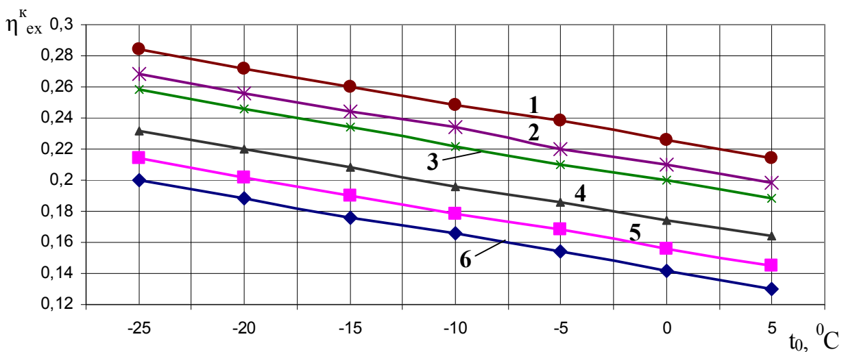
Рис. 2. Значения эксергетического КПД котла: 1 – t_{ncв}/t_{ocв} = 130 / 70^\circ\text{C} ; 2 – 120/60; 3 – 100/60; 4 – 90/50; 5 – 80/40; 6 – 70/40; t_{ncв}, t_{ocв} – температура прямой и обратной сетевой воды соответственно
