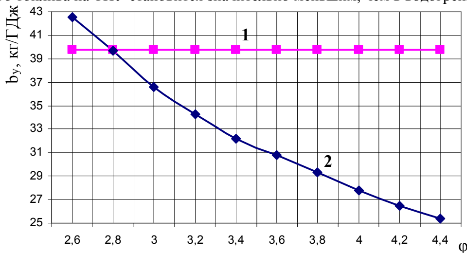
Рис. 1. Текущие значения b_y
