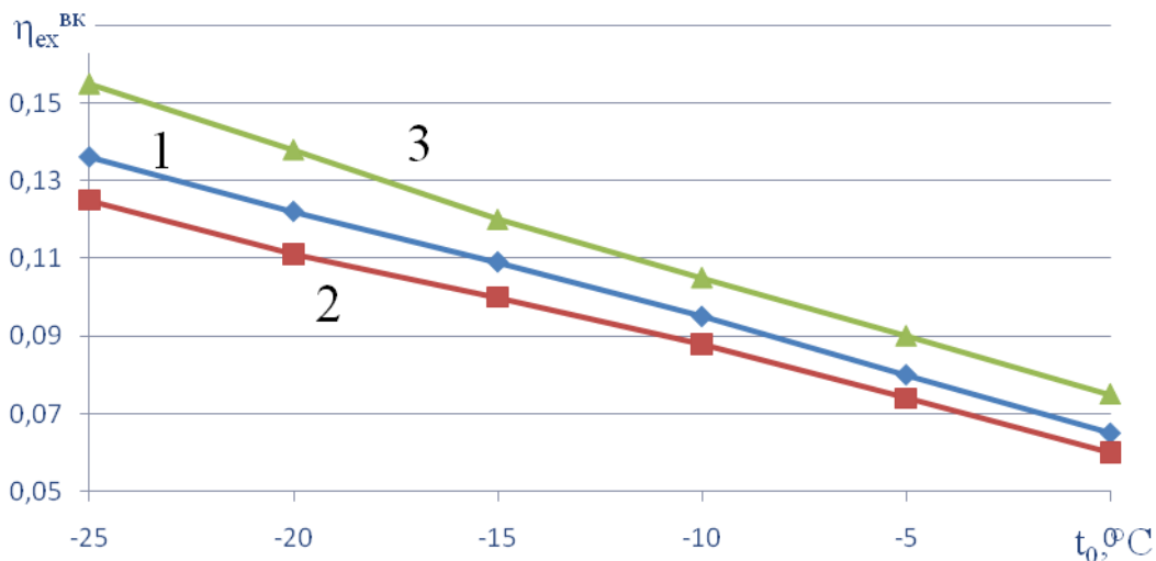
Рис. 5. Значения эксергетических КПД в системах теплоснабжения от водогрейной котельной: 1 – \eta_k = 0,9 , T_{cp}^p = 328 К; 2 – \eta_k = 0,85 , T_{cp}^p = 328 К; 3 – \eta_k = 0,9 , T_{cp}^p = 318 К
