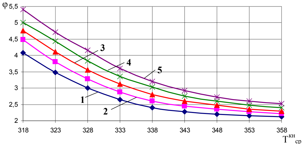
Рис. 3. Значения \varphi : 1 – T_{cp}^u = 278 К; 2 – 283; 3 – 288; 4 – 293; 5 – 298
