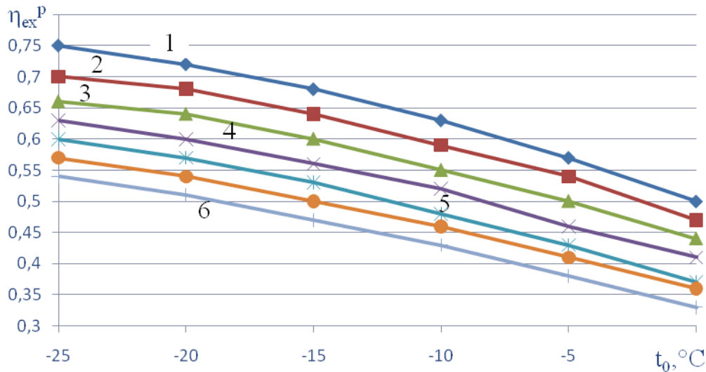
Рис. 4. Зависимости \eta_{ex}^p = f(t_0) : 1 – T_{cp}^p = 303 К; 2 – 313; 3 – 323; 4 – 328; 5 – 343
