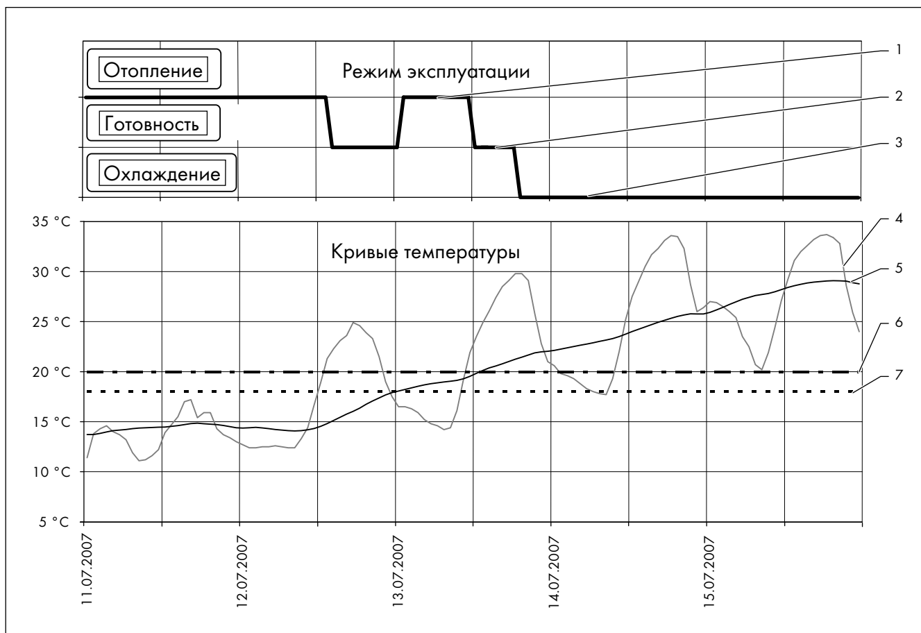
3.5 Пример зависимого от температуры наружного воздуха переключение между отоплением и охлаждением
